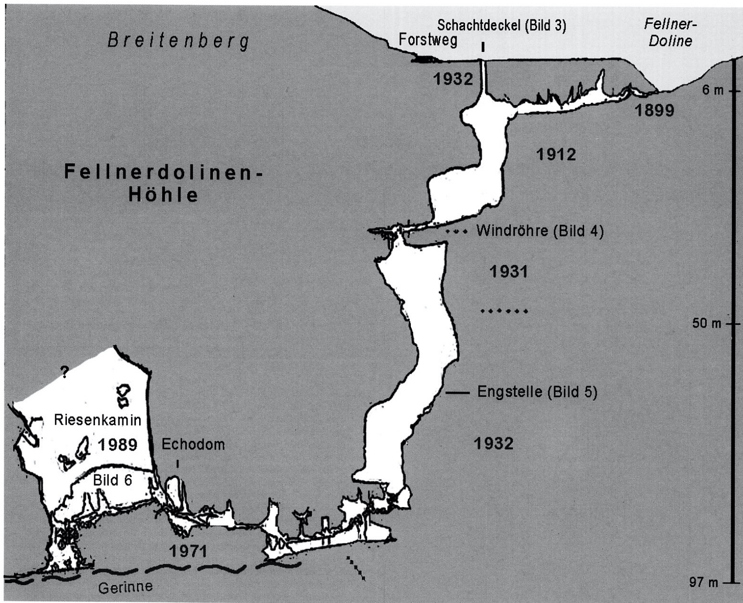
Bild 2: Aufriss der Fellnerdolinen-Höhle (nicht überhöht). Höhlengang-Vermessung durch Speläo-Club Frankenalb 1971, ergänzt durch Andreas Hartwig 2003.
