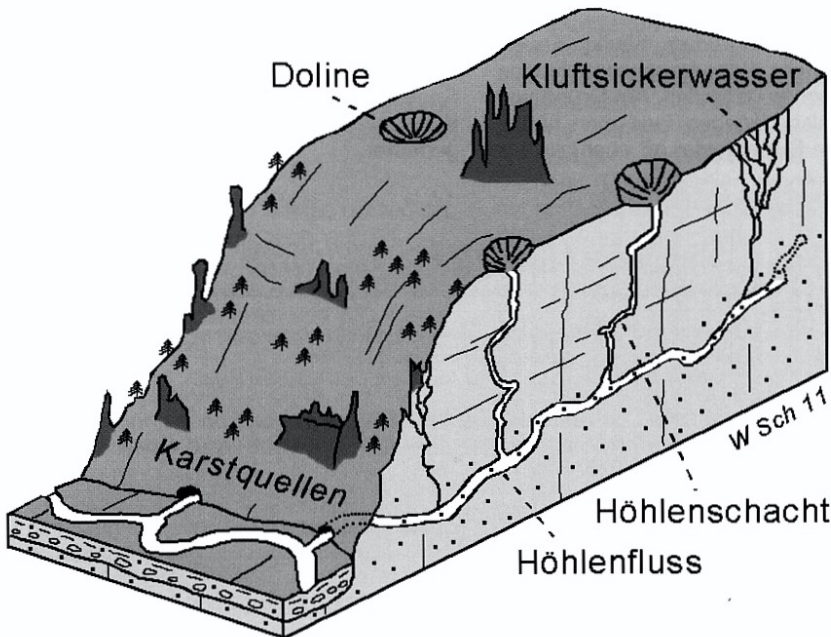
Bild 1: Schema Doline – Höhlenschacht – Höhlenfluss – Karstquelle. Gepunktet = porenwassererfüllter Teil des Karstgebirges.
