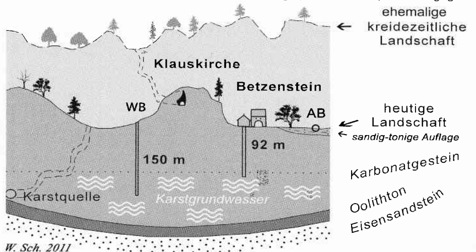
Bild ❶ – Schematische Skizze der ehemaligen und heutigen Landschaft und ihrer Wasserhältnisse um Betzenstein (unmaßstäblich) AB = Alter Brunnen. WB = Heutige Wasserversorgung durch die 150 m-Bohrung der Wassergruppe Betzenstein.
