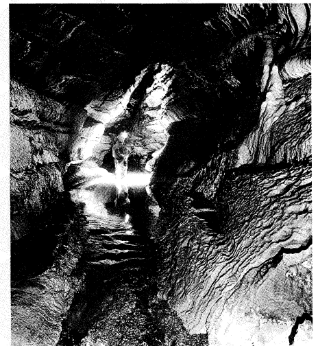
Bild 4 – Unterirdischer Wasserlauf der Mühlbach-Quellhöhle bei Dietfurt/Altmühl.
