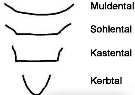
Bild 2: Taltypen des Hummerstals.
