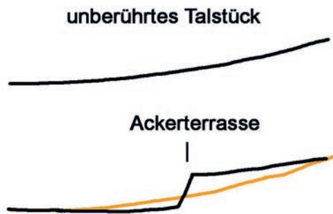
Bild 6: Entstehung der Ackerterrassen (schematisch).
